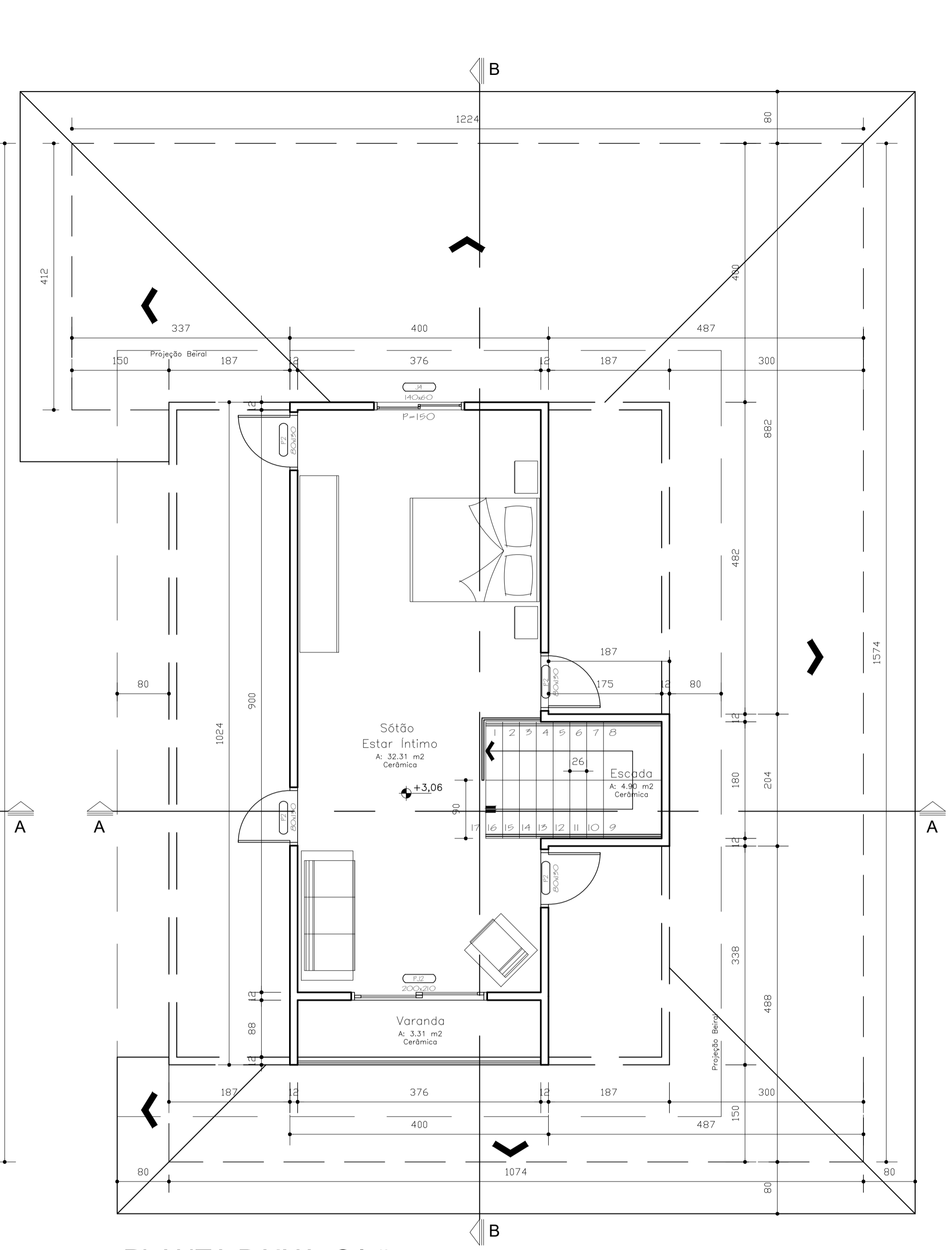
PLANTA BAIXA_Sótão Esc. 1:50
