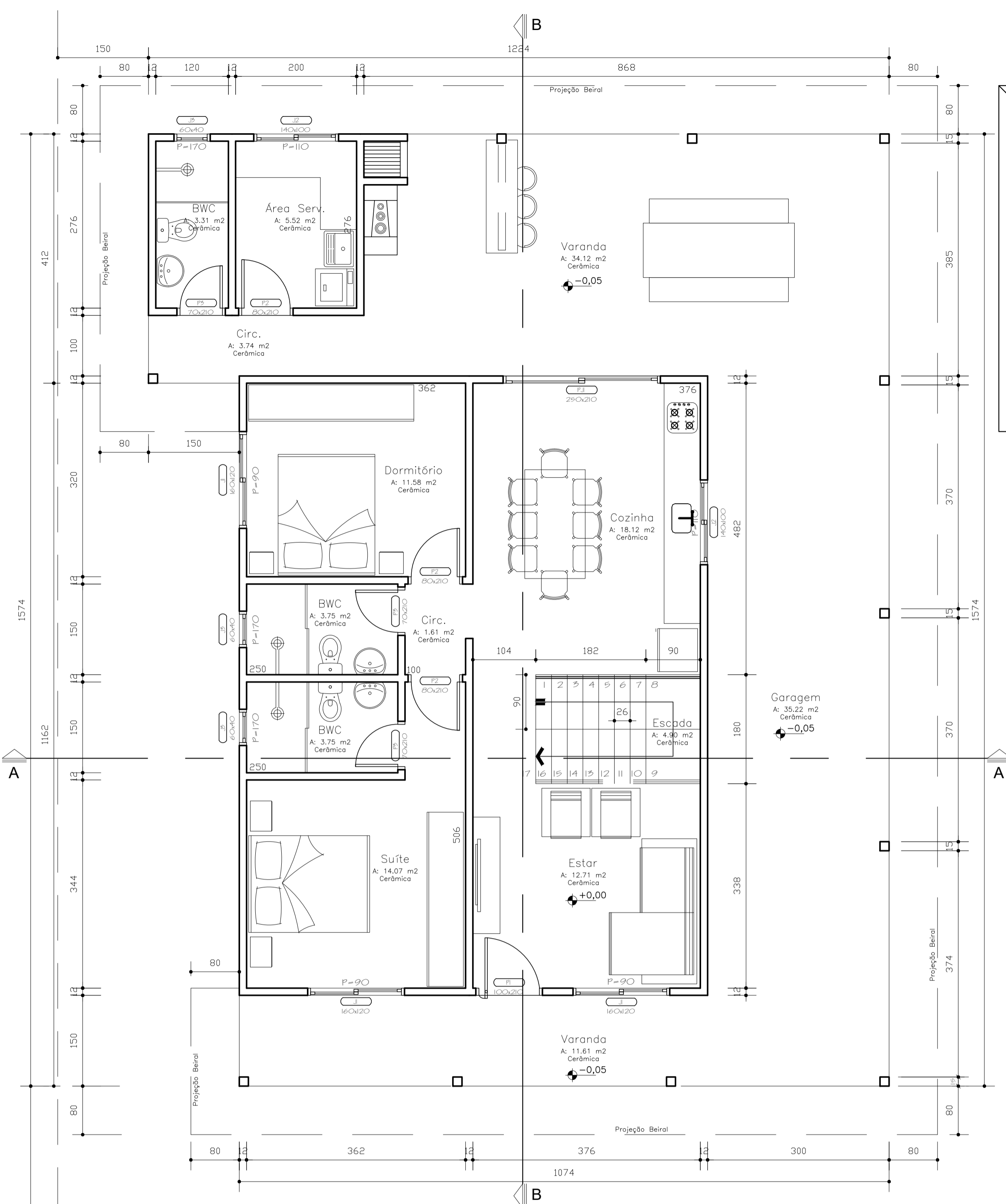
PLANTA BAIXA_Térreo Esc. 1:50
